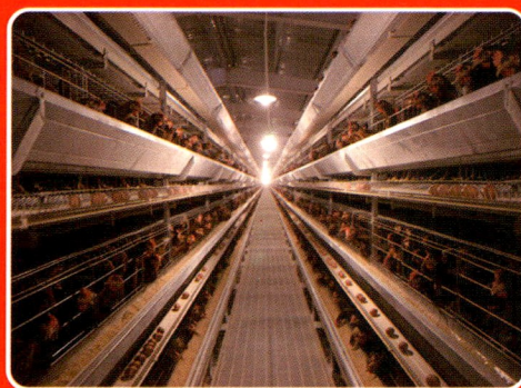
层叠式自动化蛋鸡饲养设备
