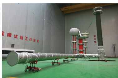
特高压环保管道样机型式试验
