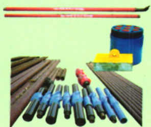
钻铤、钻杆、辅助工具、强磁打捞器、绳索取心液动锤
