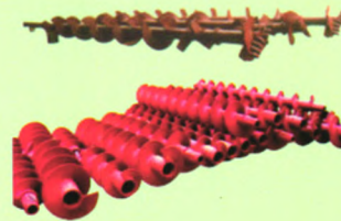
长螺旋转钻具及SMW工法钻具
