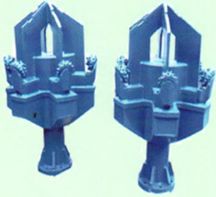
煤矿救援孔用扩孔牙轮钻头
