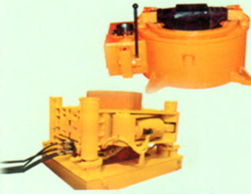
Lz500转盘和用于 全套管钻进的 拔管机
