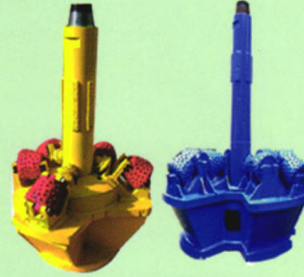
煤矿钻井用反井钻头
