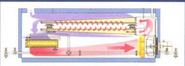
热风循环示意图 独特平顶结构, 使烘箱内无滴油现象。
