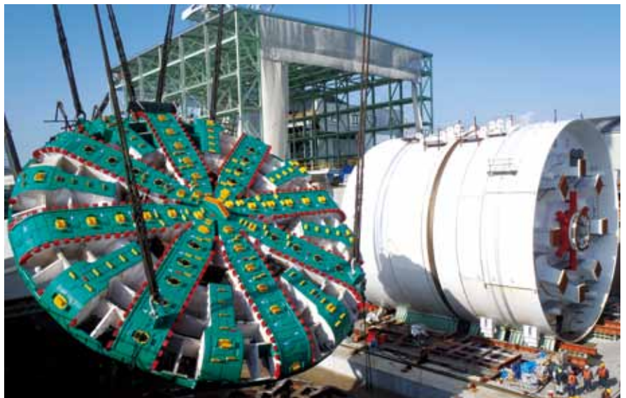
100 拯救地下巨无霸“伯莎”
