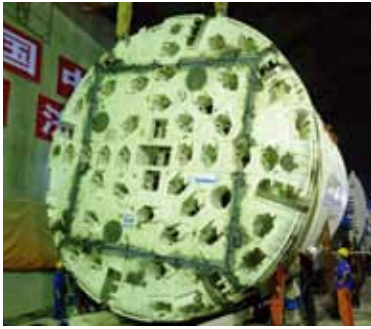
104 引汉济渭秦岭隧 道岭南项目TBM 洞内组装
