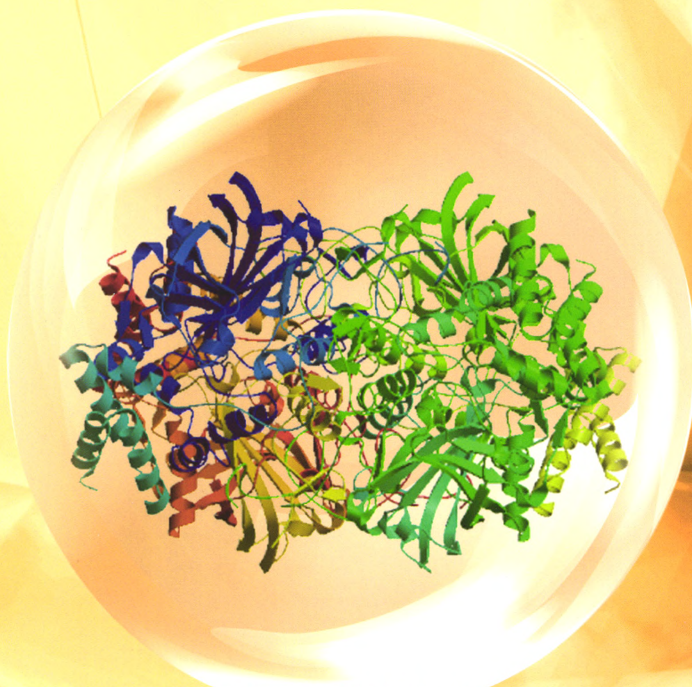
陆稻OsCATB-lh编码蛋白三级结构 (内文第 109 页)
