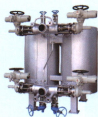
预聚物过滤器
