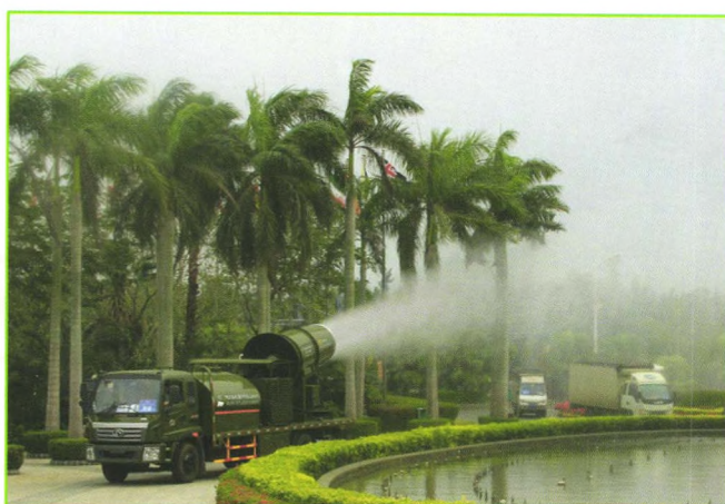
一种控制PM 2.5 空气质量超标的移动式水雾降尘机车 （专利号：201220226287.6）
