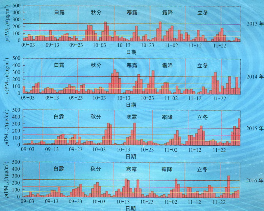
2013—2016年北京秋季(9—11月) \rho(\text{PM}_{2.5}) 逐日变化趋势
