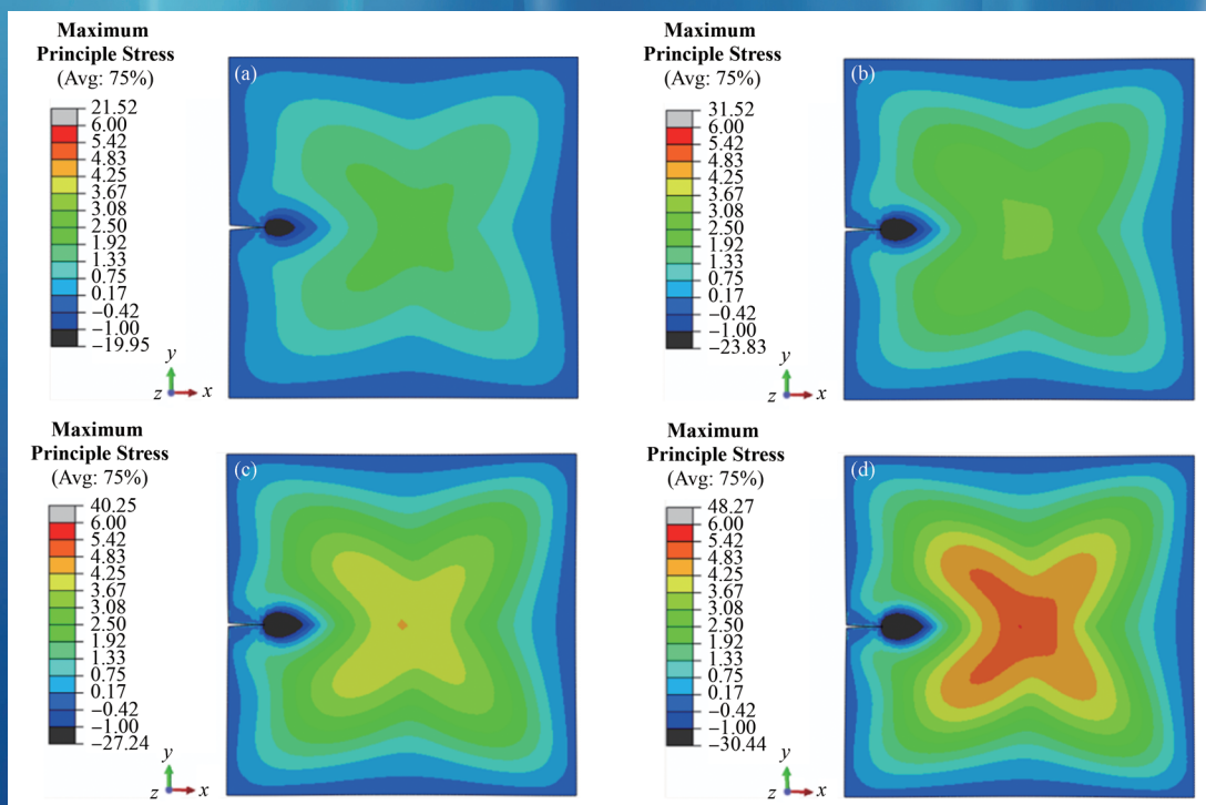
V型凹口半宽度0.5 mm构件最大主应力分布 (P.070601) (a) 辐照梯度为10%, (b) 辐照梯度为15%, (c) 辐照梯度为20%, (d) 辐照梯度为25%
