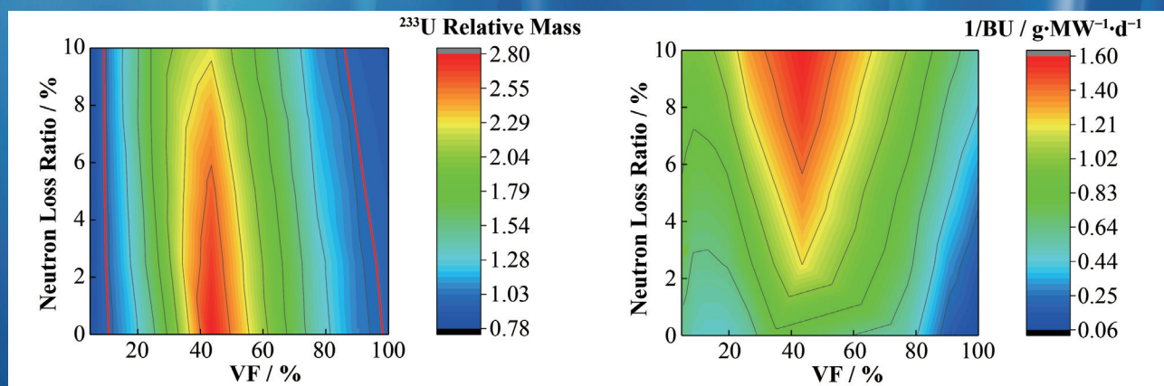
20年燃耗时 233 U的自持比(左)和对钚的依赖(右) (P.030601)
