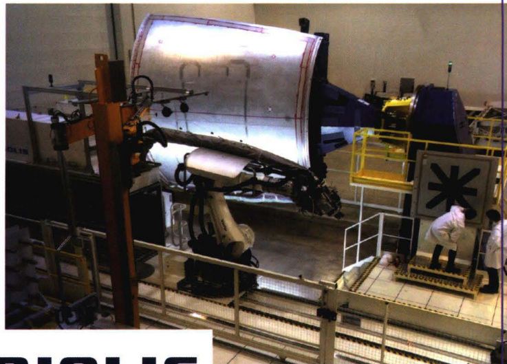
法国 STELIA 的 A350 前机身壁板批产
