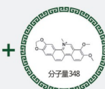
白屈菜红碱
