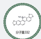
血根碱
