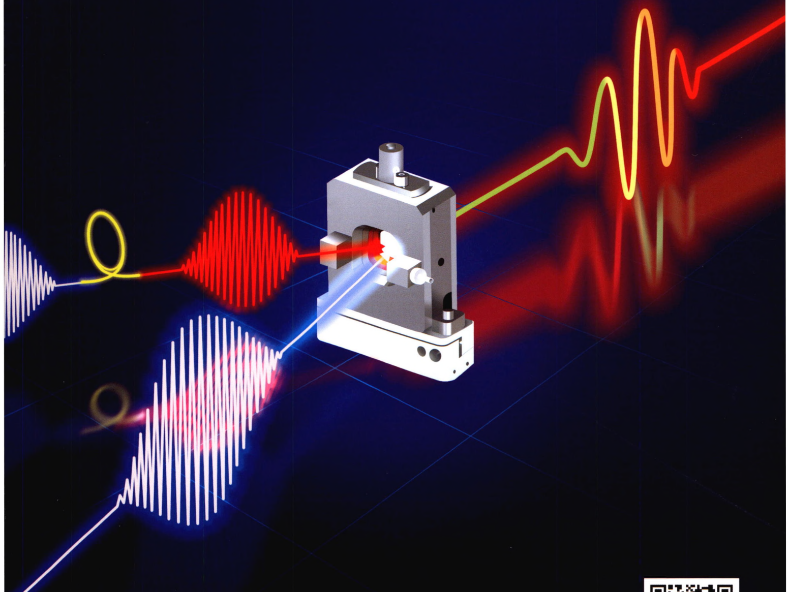
封面图片：超快光纤激光驱动的长波中红外飞秒脉冲光源 / 刘洋
