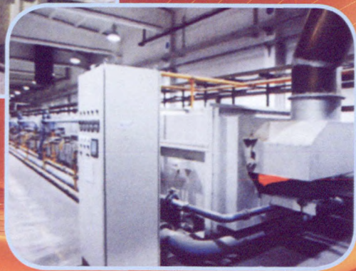
中丝预处理生产线
