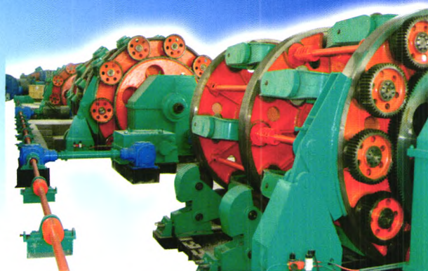
KL(12+30+30)/630 大型筐篮串联机组
