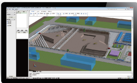
△ 土方开挖模拟及方案设计
