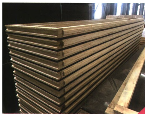
装配可拆式钢筋桁架楼承板
