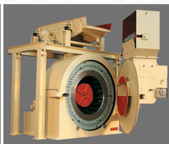
BX4614/5刨片机
