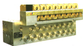
SAC型电液控制系统
