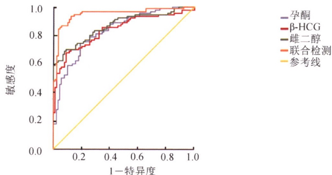
图5 血清孕酮、 \beta -HCG与雌二醇单项与联合检测早期先兆流产的ROC曲线
