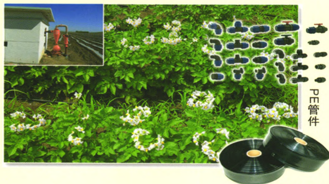
8DWG-50型滴灌设备
