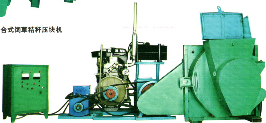
9KWH-45型柴油机驱动组合式饲草秸秆压块机
