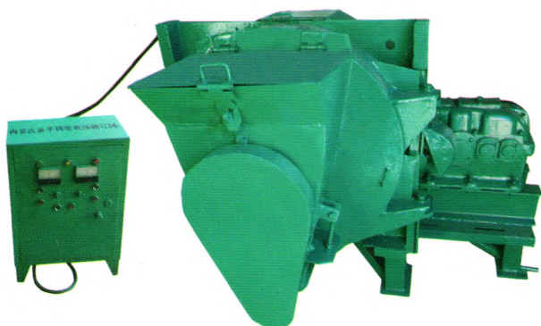
9KWH-20型电驱动组合式饲草秸秆压块机
