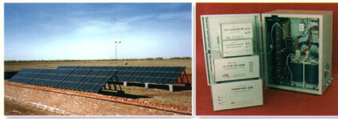
风光互补村落供电系统
