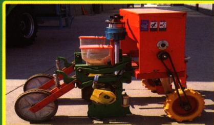
七膜十四行 配套动力：180马力以上 总成膜宽：700mm 纯小时生产率：12亩
