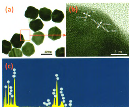
(a) 反应温度为315°C时合成的NaLuF4透射电镜照片; (b) 反应温度为315°C时合成的NaLuF4高分辨透射电镜照片; (c) NaLuF4: 20%Yb 3+ , 2%Er 3+ 元素分析谱
