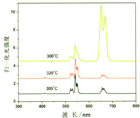
图4 300、305与320°C制备NaLuF4纳米晶的发射光谱
