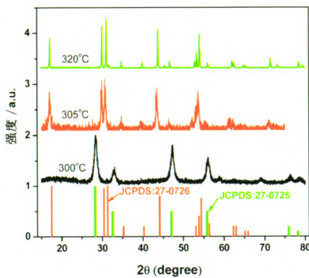
图3 反应温度为300、305与320°C时合成的NaLuF4的XRD图谱
