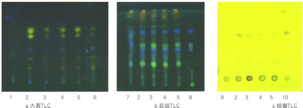
1:缺大黄阴性对照；2~5:供试品；6:大黄对照药材；7:缺前胡阴性对照；8:前胡对照药材；9:缺槟榔阴性对照；10:槟榔对照药材
