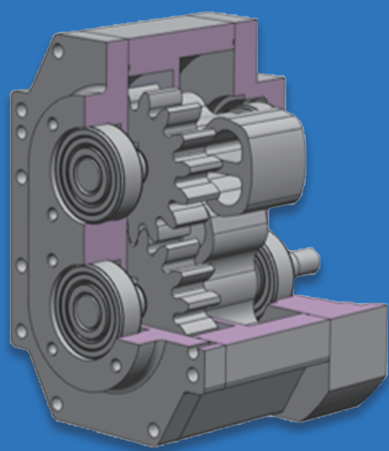
凸轮式氢气循环泵三维模型
