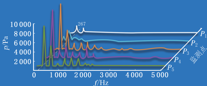
监测点压力脉动频域特性
