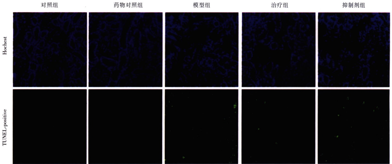
图2 激活GLP-1R对肾脏细胞凋亡的影响(TUNEL, ×200)
