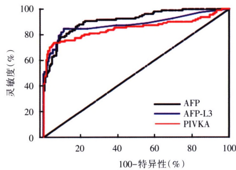
图2 血清AFP、PIVKA-II及AFP-L3浓度诊断肝癌的ROC分析
