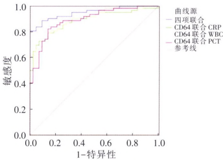
图 1 CD64 指数、CRP、WBC 及 PCT 诊断重症患者感染的 ROC 曲线
