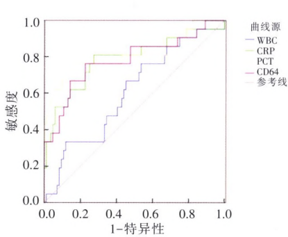
图 2 CD64 指数、CRP、WBC 及 PCT 预测重症患者预后的 ROC 曲线
