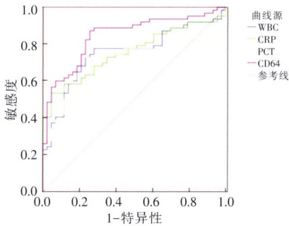
图 1 CD64 指数、CRP、WBC 及 PCT 诊断重症患者感染的 ROC 曲线
