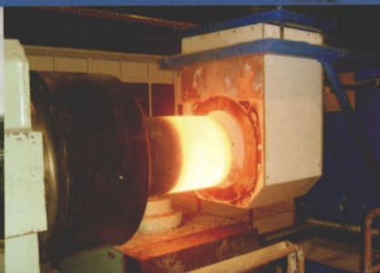
热旋压收口
