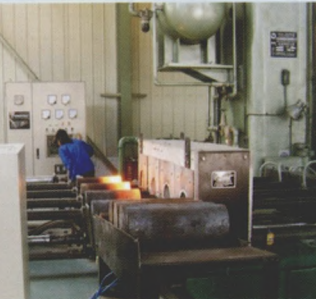
弹体毛坯端部加热
