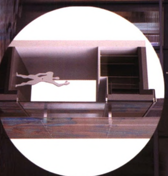
1:5 节点的造模型研究 11m 超大单曲弯钢化中空三银LOW-E玻璃
