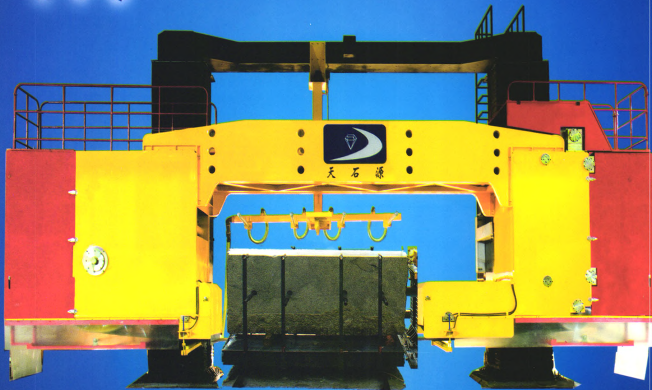
TSY-MW42U 多绳锯机
