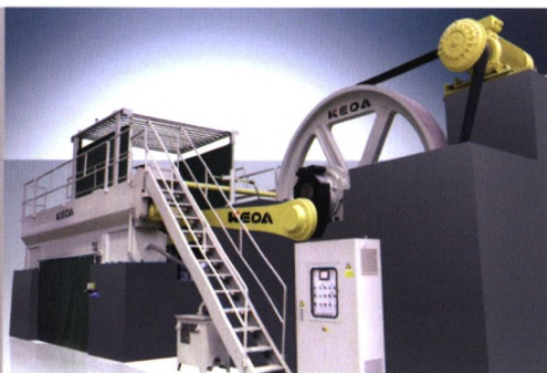
大理石静压排锯
