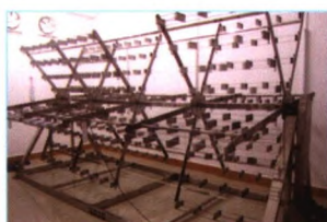
蚕种催青机
