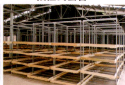
活动蚕台
