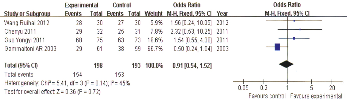
图 1 两组治疗有效率的森林图
