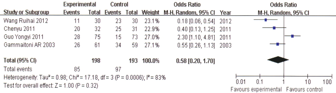
图 2 两组不良反应发生率的森林图
