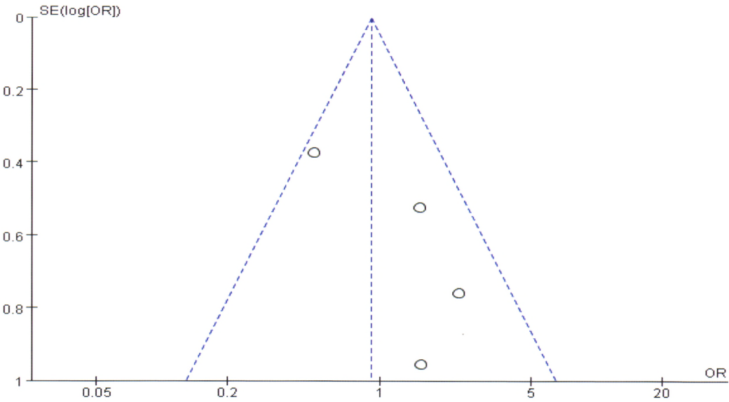
图 3 两组治疗有效率的漏斗图
