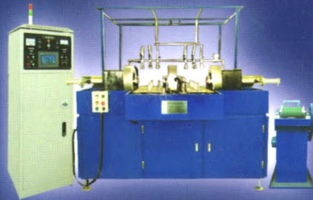
ZY-CEW-2000L 连杆专用磁粉探伤机组(自动上下料、双磁化工位)
