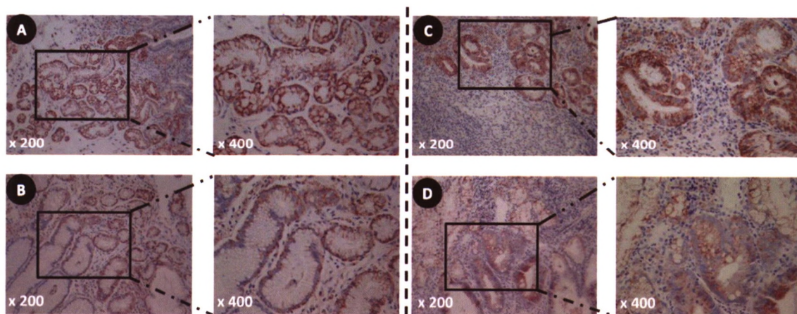
A: 对照组治疗前; B: 对照组治疗后; C: 联合组治疗前; D: 联合组治疗后 图 1 两组患者治疗前后胃组织 COX-2 表达情况比较(免疫组化染色)
