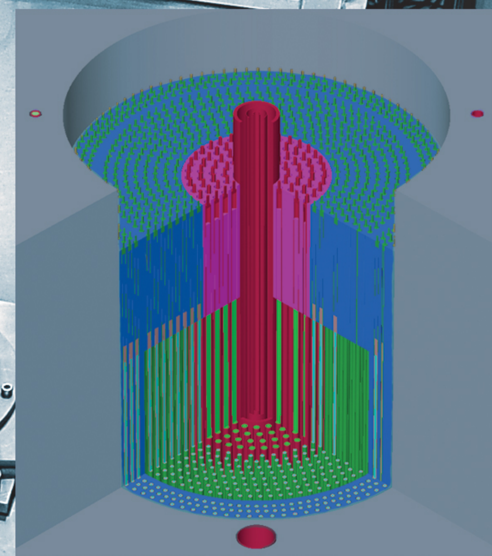
堆芯斜剖面图
