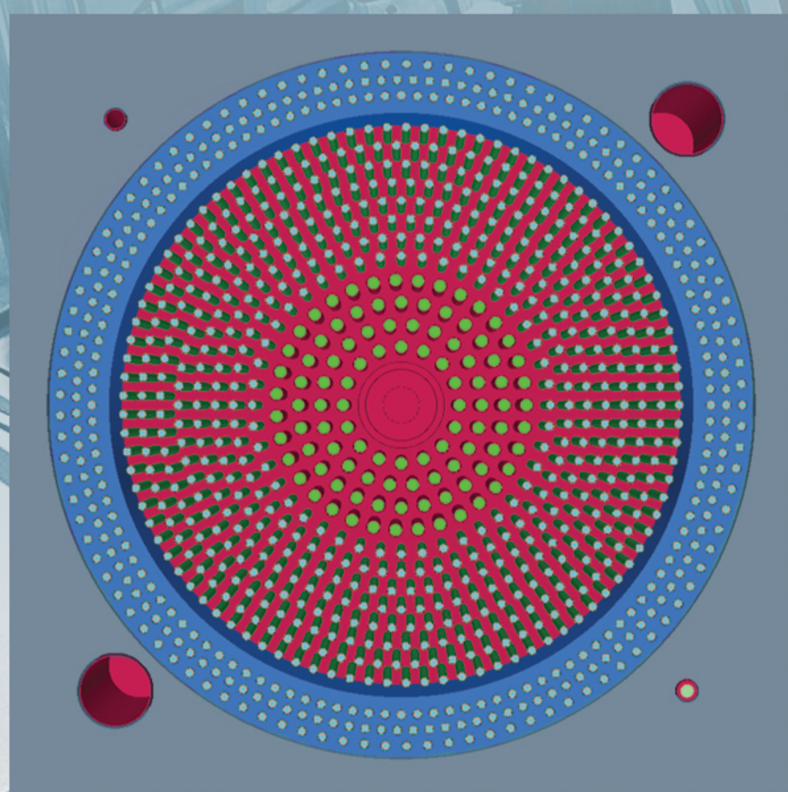
堆芯横剖面图
