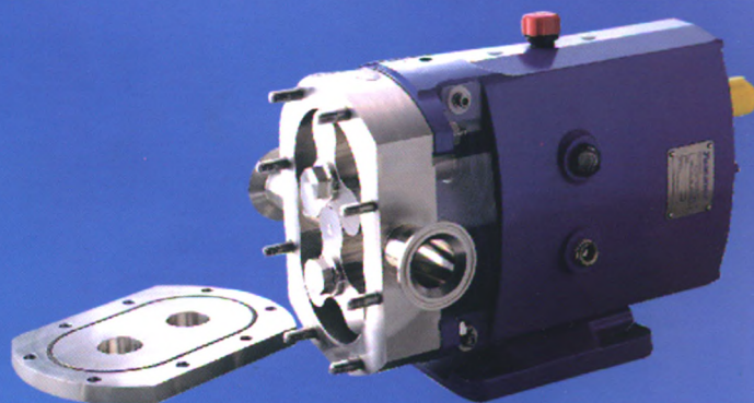
YAS 转子泵
