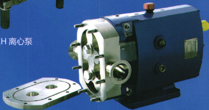
YAS 转子泵
