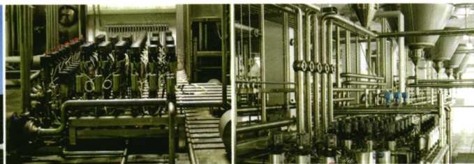
阀阵
