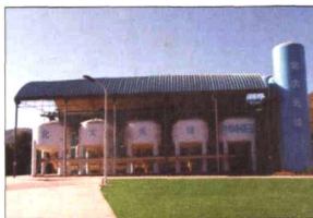
7500Nm 3 /h 变压吸附空气分离制氧装置
