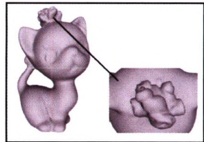
三次B样条插值的网格拼接和融合(第1901页)
