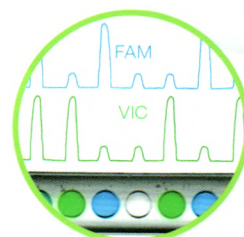
4. 报告结果
