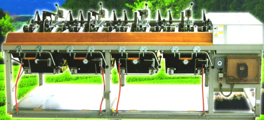
清洁化绿茶、红茶生产流水线
