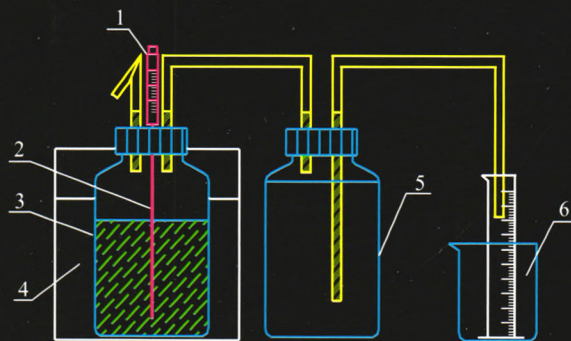
1-针筒; 2-细钢管; 3-发酵瓶; 4-恒温水浴锅; 5-沼气的收集瓶; 6-量筒
